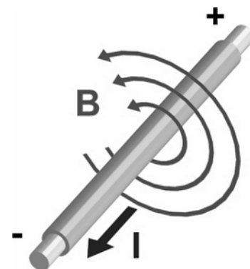
Рис. 2. Направление вектора магнитной индукции в соответствии с правилом буравчика (на рисунке изображен прямой провод с током; ток I , протекая через провод, создает магнитное поле B вокруг провода).
