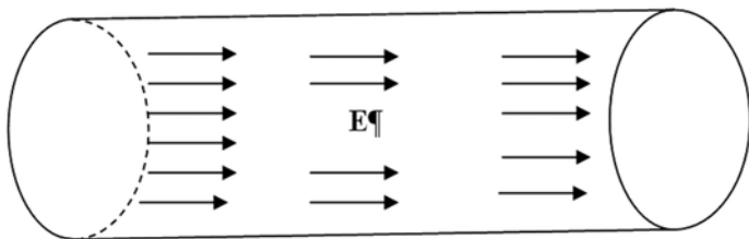
Рис. 3. Участок провода с током.
