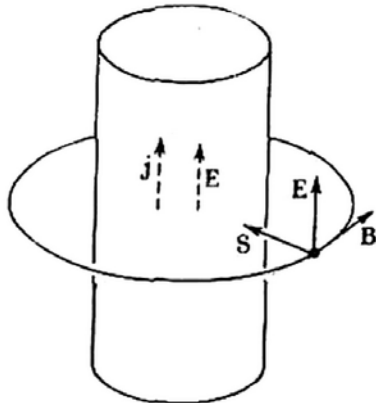
Фиг. 27.5. Вектор Пойнтинга S вблизи провода с током.
