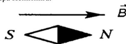
Рис. 1. Направление вектора магнитной индукции
